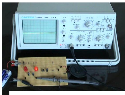
图 2-11 示波器观看波形
